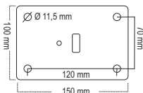
Fußplatte für Poller Ø 60-89 mm 8 mm dick
