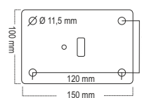
Fußplatte für Poller Ø 60-89 mm 8 mm dick
