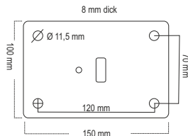
Abmessung der Fußplatte für Pfosten 70x70, Ø 76 und 89 mm
