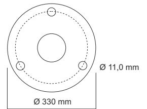
techn. Daten der Fußplatte für Pfosten Ø 254 mm 6 mm dick
