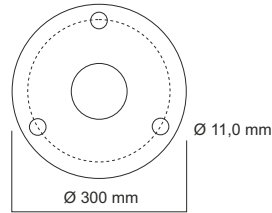
techn. Daten der Fußplatte für Pfosten Ø 219 mm 6 mm dick
